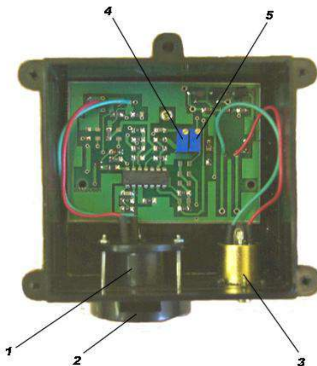
Рис.3. Датчик СИГМА-03.ДЭ со снятой крышкой. 1 - Сенсор оксида углерода электрохимический; 2 – фланец; 3 – вилка; 4 – потенциометр регулировки усиления; 5 – потенциометр регулировки начального ток.
